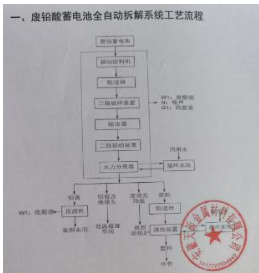
工艺流程图
